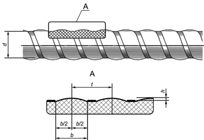
Рисунок А.3 — Конфигурация и параметры периодического профиля АКП по форме 3ф
